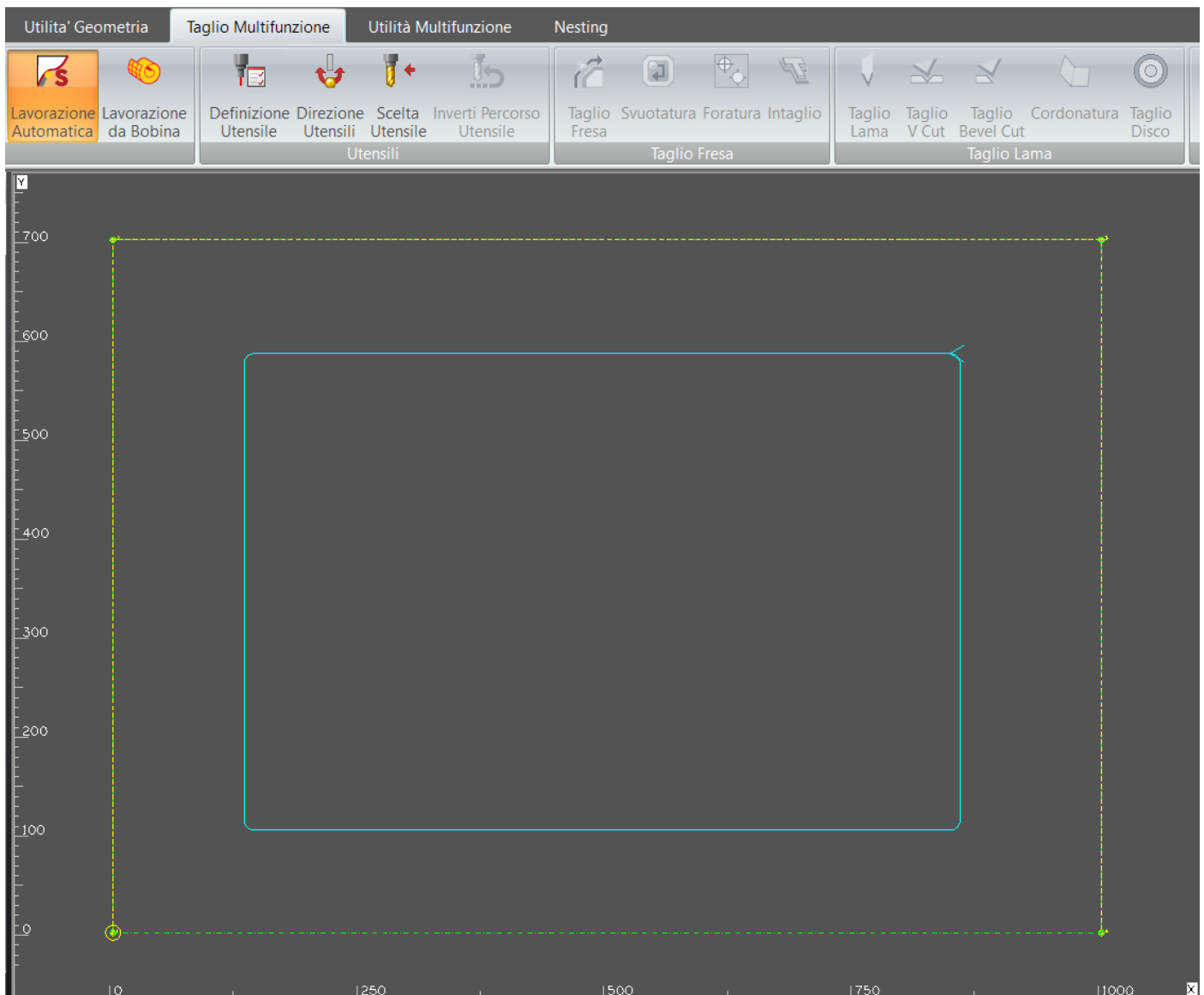
Figura 5: Una volta controllati tutti i livelli e assegnati i registri applicare le lavorazioni con "lavorazione automatica" oppure applicare le lavorazioni personalizzate e poi in "Utilità Multifunzione" assegnare i registri Visiotek
